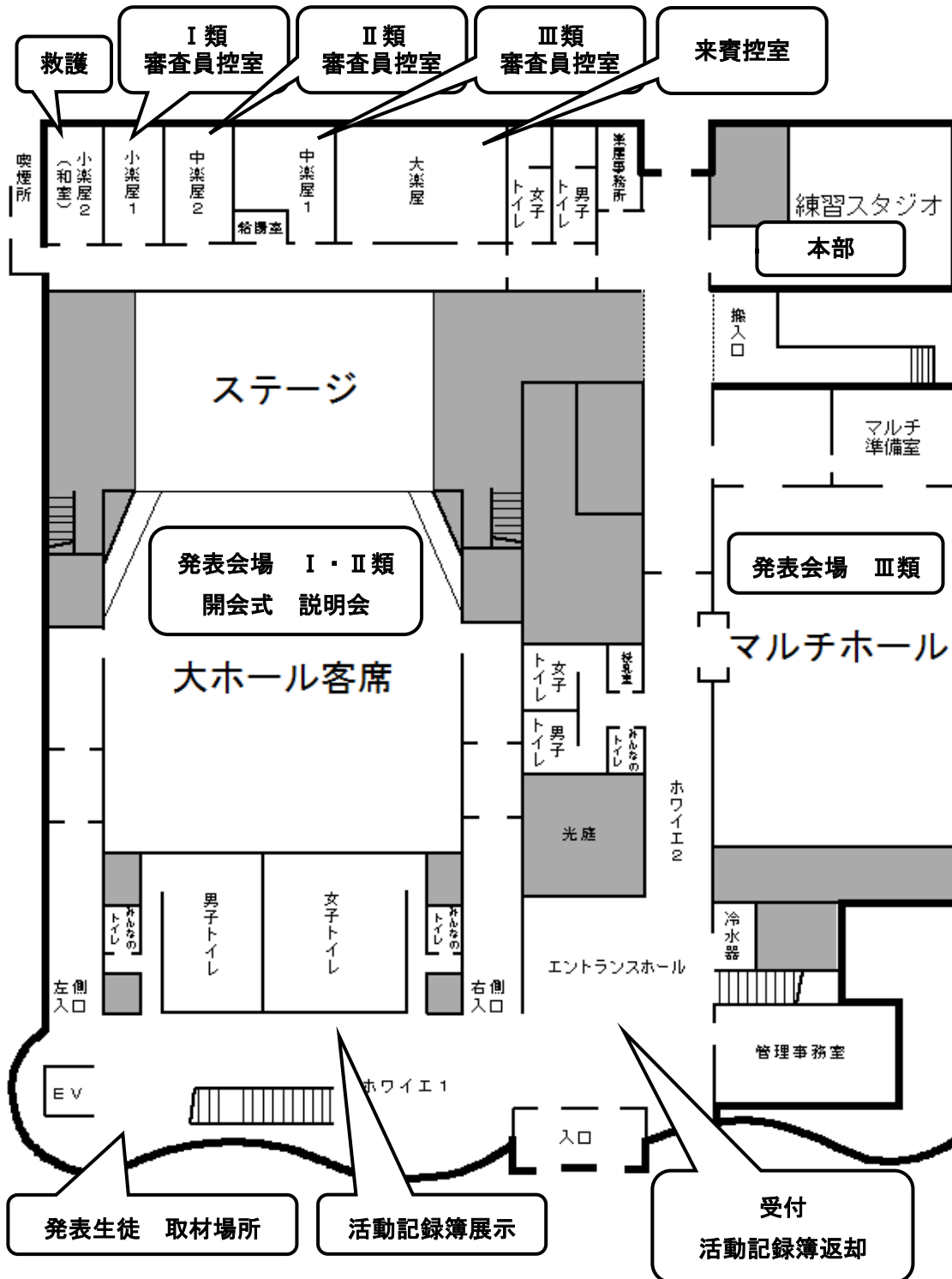
玉名市民会館ホール棟
